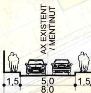
PROFIL PROPUȘ (C-C) - STRADA POEMULUI - PROPUȘ SCARA: 1/200
