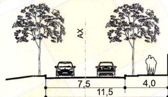
PROFIL (B-B) - STRADA GARLEI - EXISTENT / MENTINUT SCARA: 1/200
